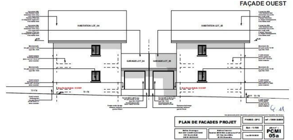
FAÇADE OUEST
