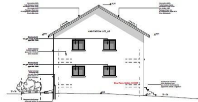
FAÇADE SUD
